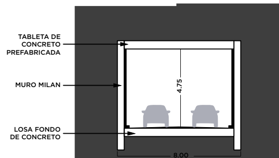
EXCAVACIÓN A CIELO ABIERTO
