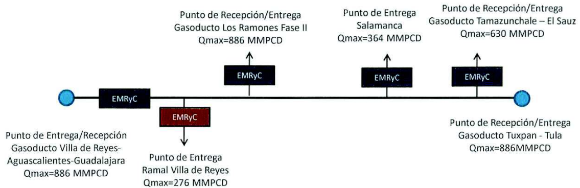
FIGURA 1 Diagrama Esquemático Sistema Tula – Villa de Reyes
