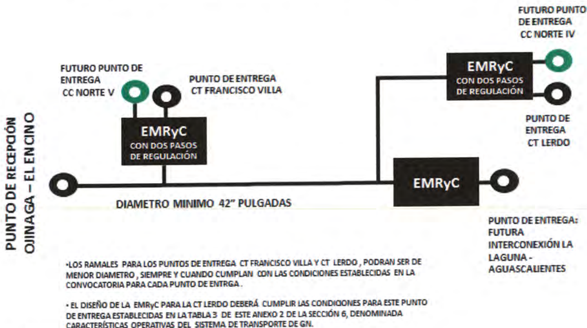
FIGURA 1 DIAGRAMA ESQUEMÁTICO DE SISTEMA EL ENCINO – LA LAGUNA
